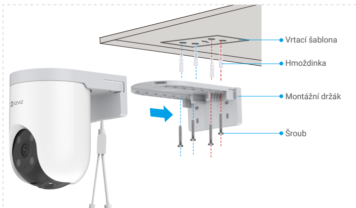
Obr. 1 Montáž na strop
